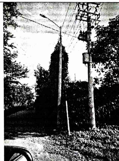
Imagen 5. Estructura de retención y luminaria LED instalada en el marco de las obras de alumbrado público rural.
